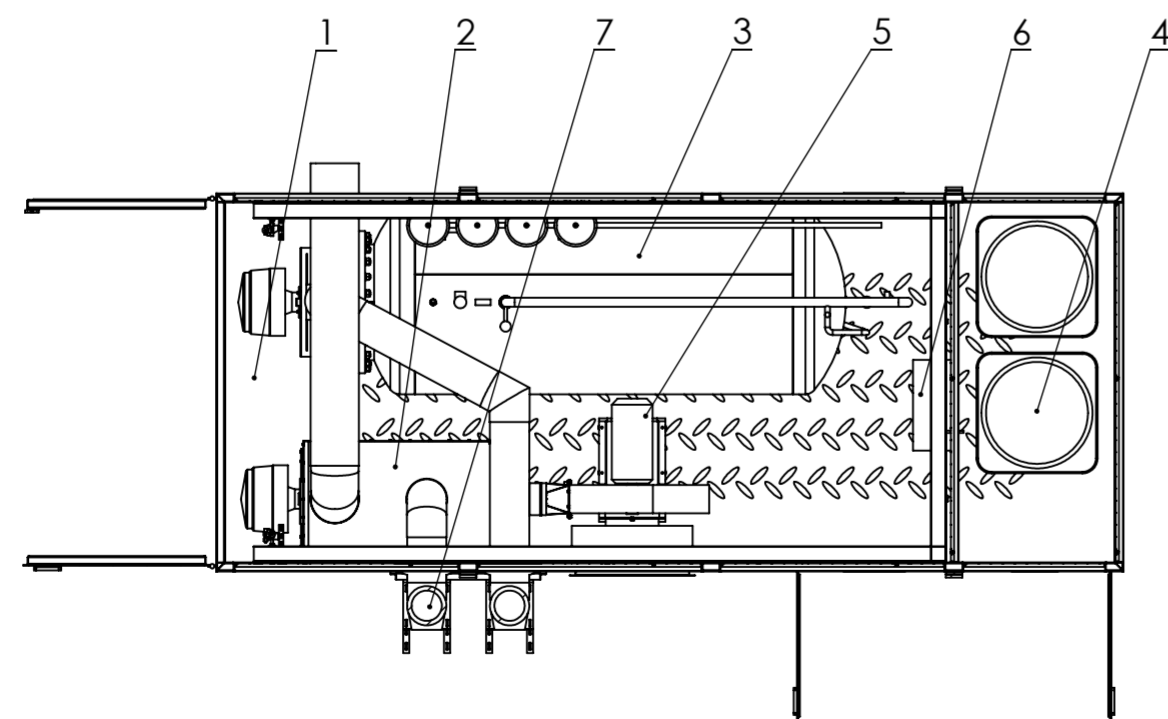
PRZEKRÓJ A-A
